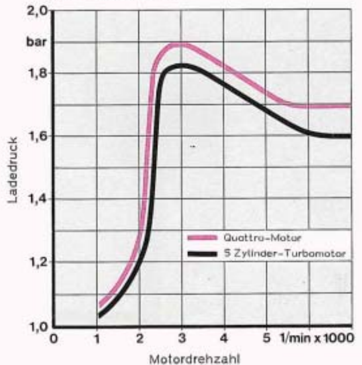
Ladedruckverlauf
